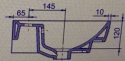
A-A' KESİTİ
