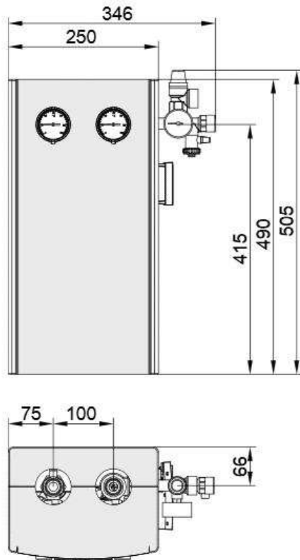
Solar-Divicon
