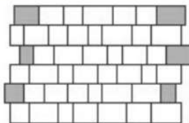
Verlegeschema Reihenverband (auch Maschinenverlegung)
