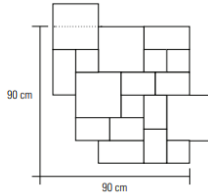
M 403: Verlegemuster aus Liefereinheit umgruppiert
